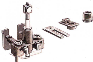
4555 B 2,90 DM Weichenlaternensatz zum Unterflurantrieb
